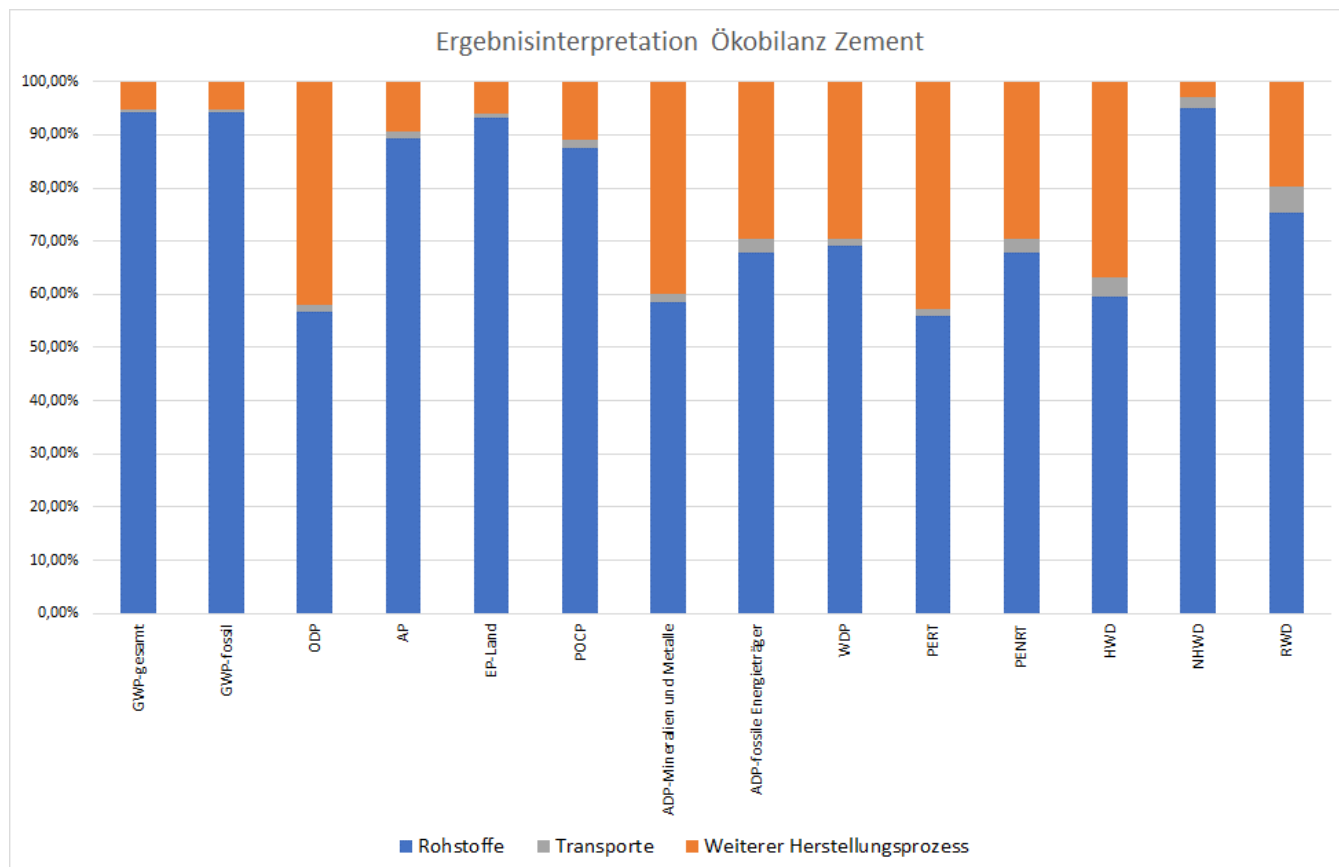
Abbildung 4: Dominanzanalyse Zementherstellung Durchschnittszement CEM II/B 32,5 N, 32,5 R, 42,5 N und 42,5 R
