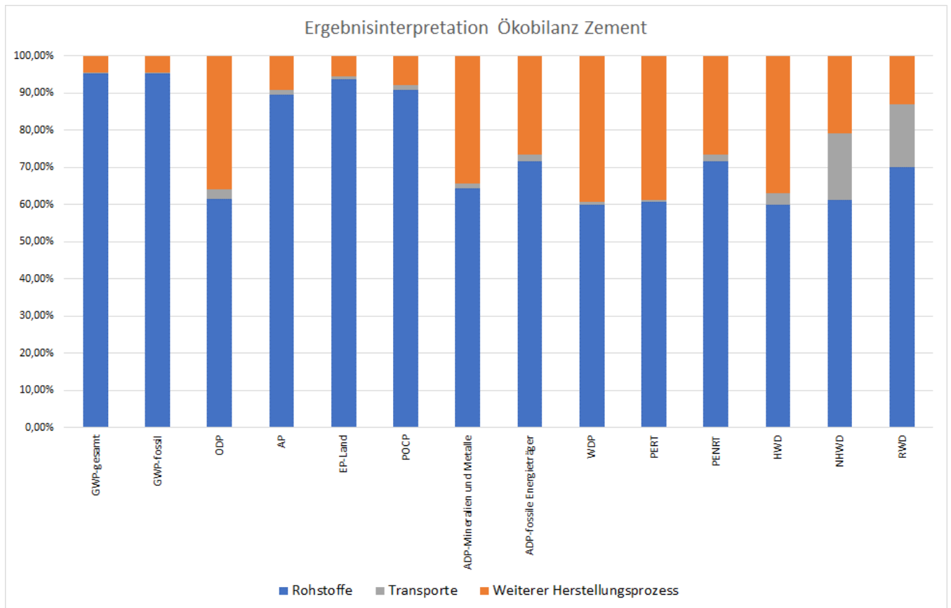
Abbildung 4: Dominanzanalyse Zementherstellung Kirchdorfer LEOcem CEM II/C-M (S-LL) 42,5 N
