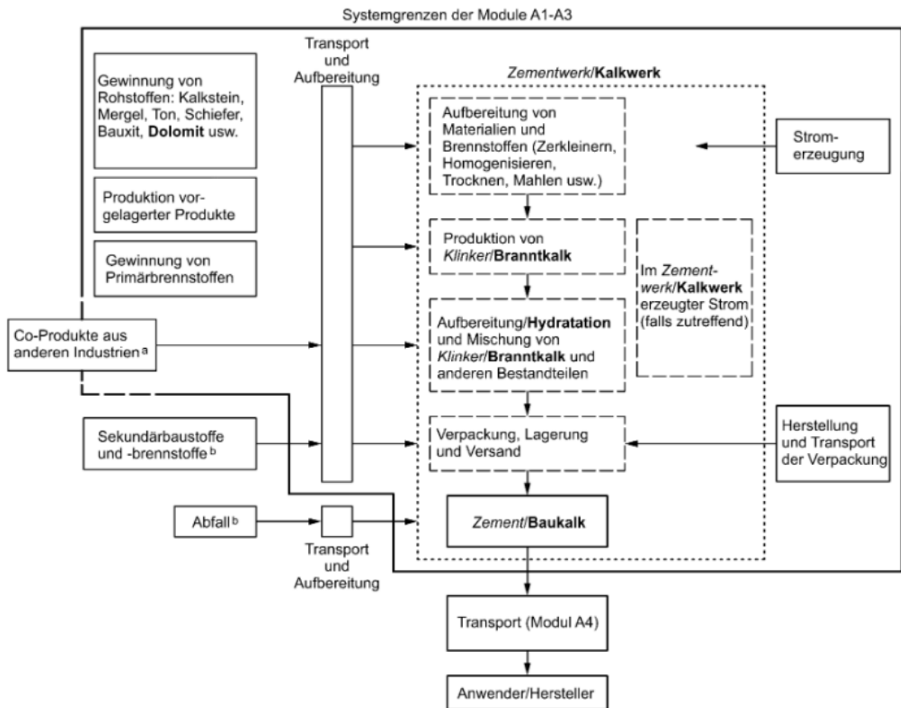
Abbildung 2: Systemgrenzen der Zementproduktion nach ÖNORM EN 16908 [6]
